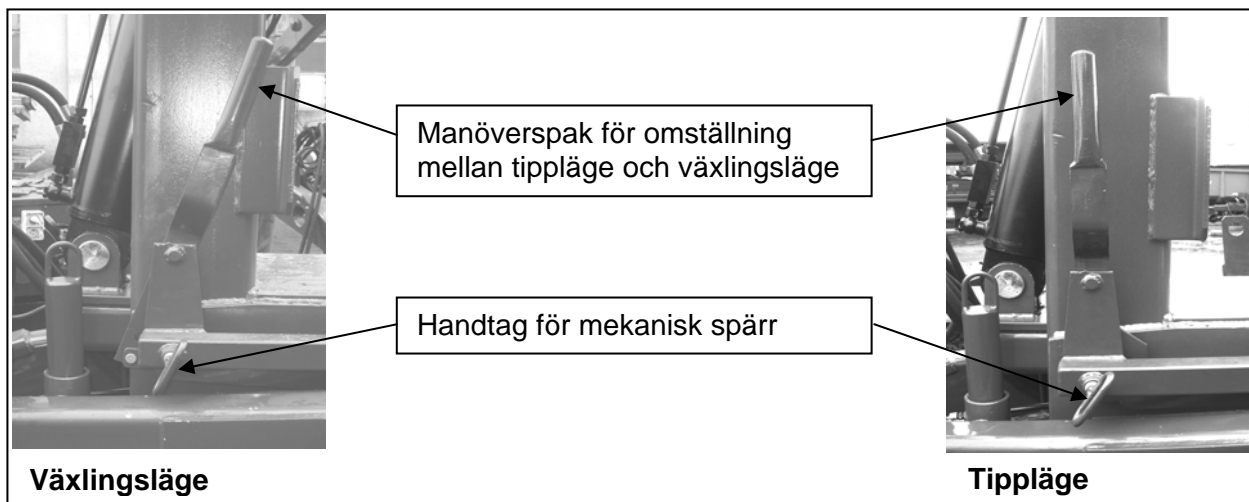
Bild 7 – Manöverspak växling/tipp
