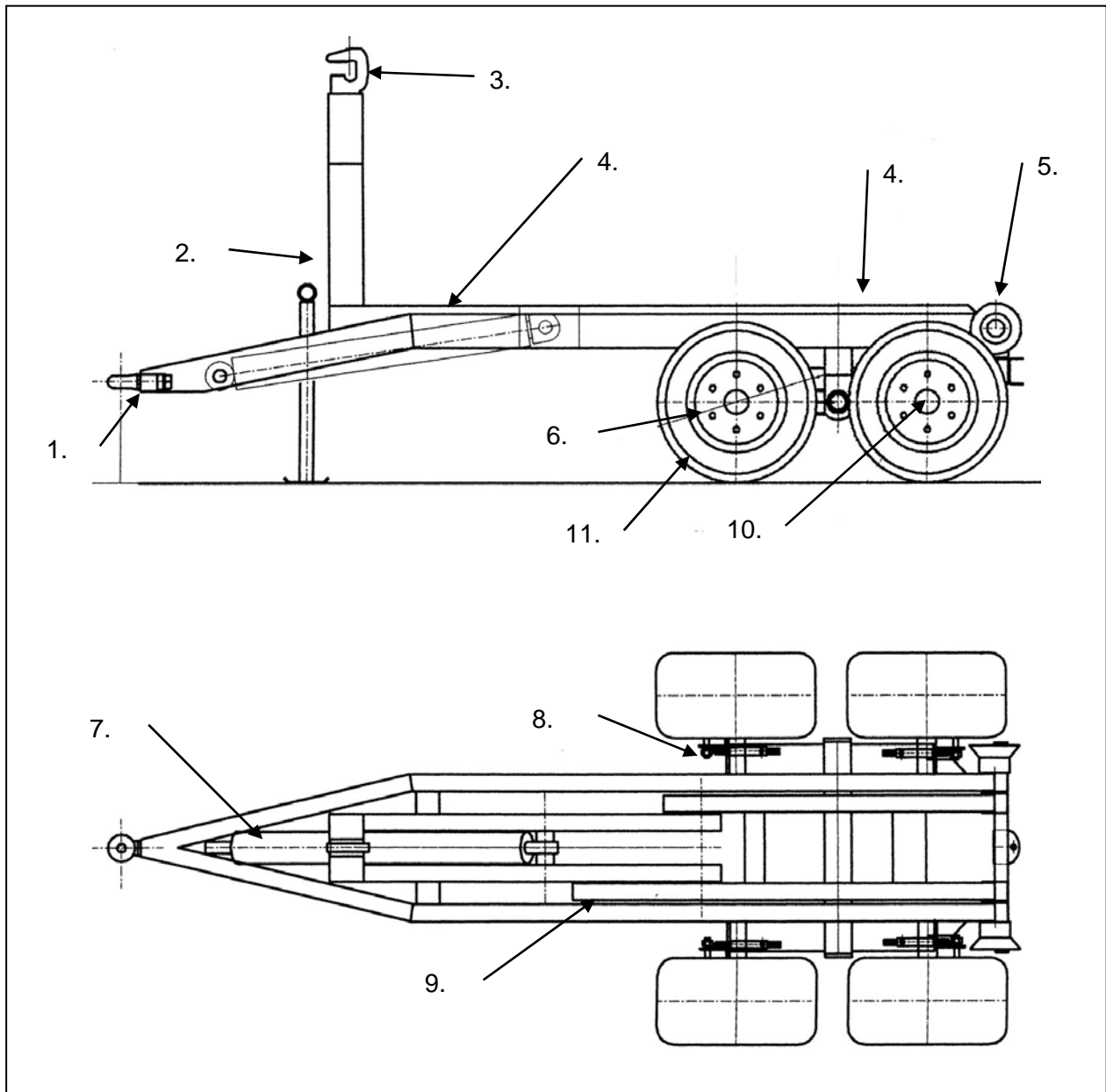
Fig. 3 - Underhållsschema
