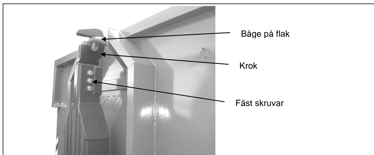
Bild 5 – Justerbar krok
