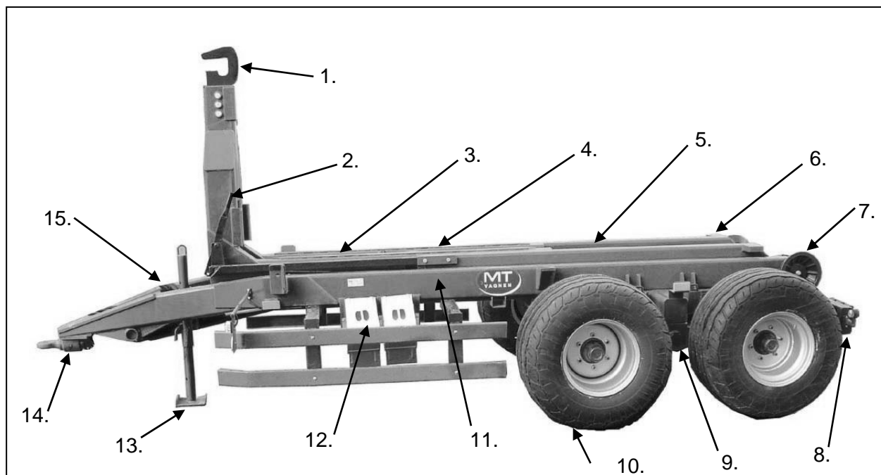
Bild 1 - Underrede och ram (Bilden visar MT8-12)
