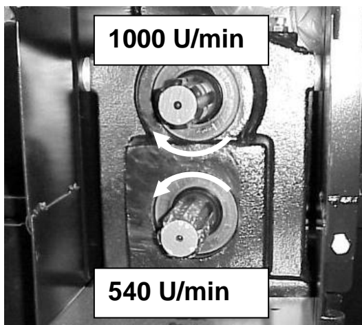
Drehzahl und Drehrichtung für Zapfwellenenden 1-3/4"
