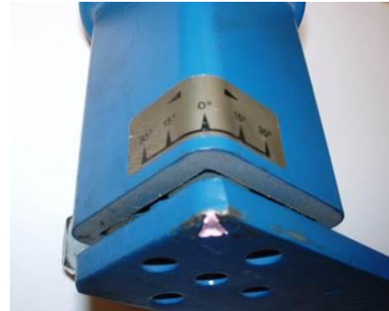
Gradanzeiger des Spannanzeigers, ab Werk auf 15 Grad voreingestellt
