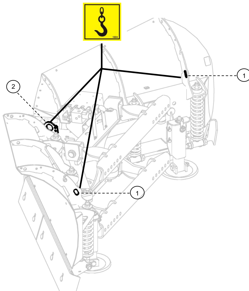
Bild.22: Lyftanvisning
