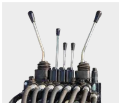
Mekaaninen venttiilipaketti 4 XY-toimintoa ja loput suorina toimintoja.
