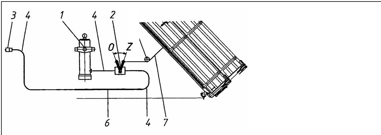
Bild 3: Hydraulschema över tippbegränsningsventil av flaket
