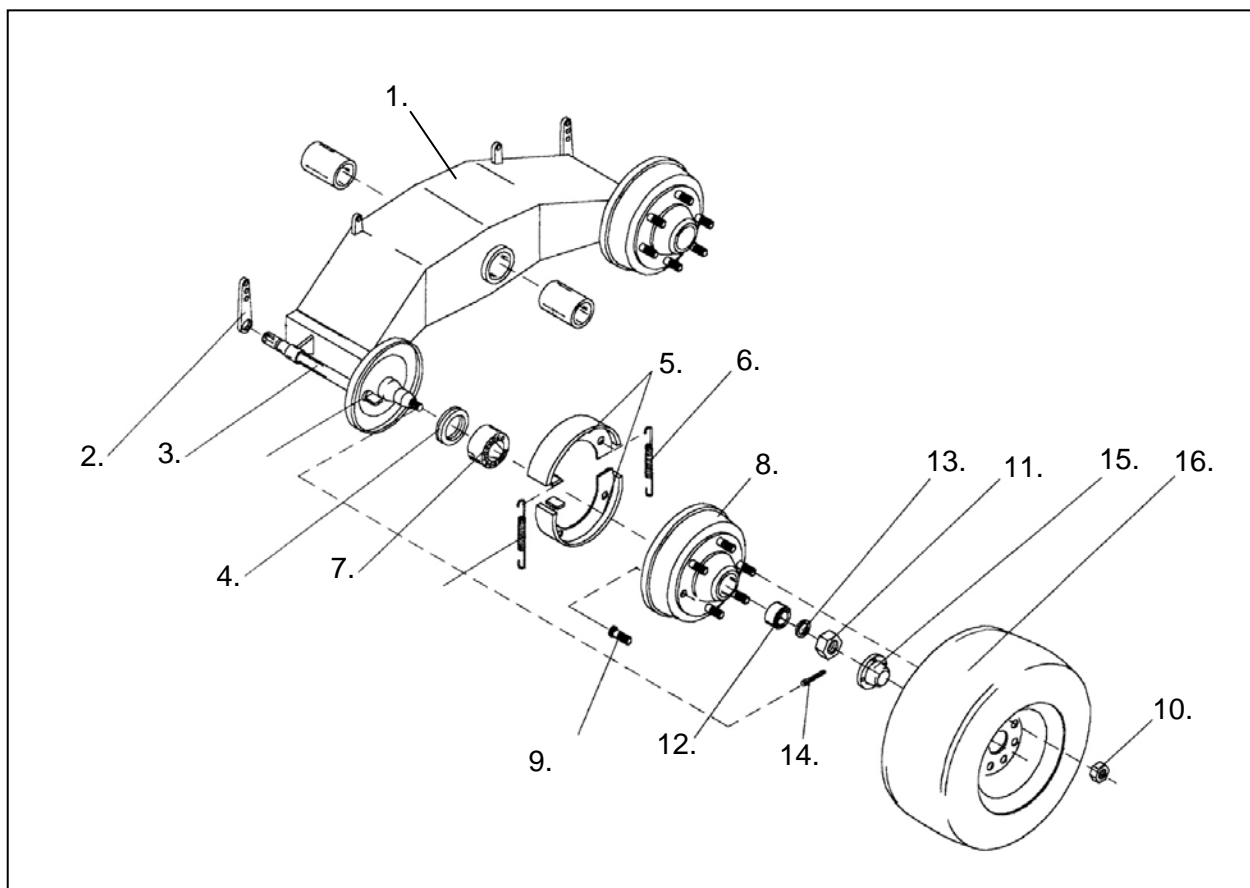
Fig. 2 - Bromsar och axlar
