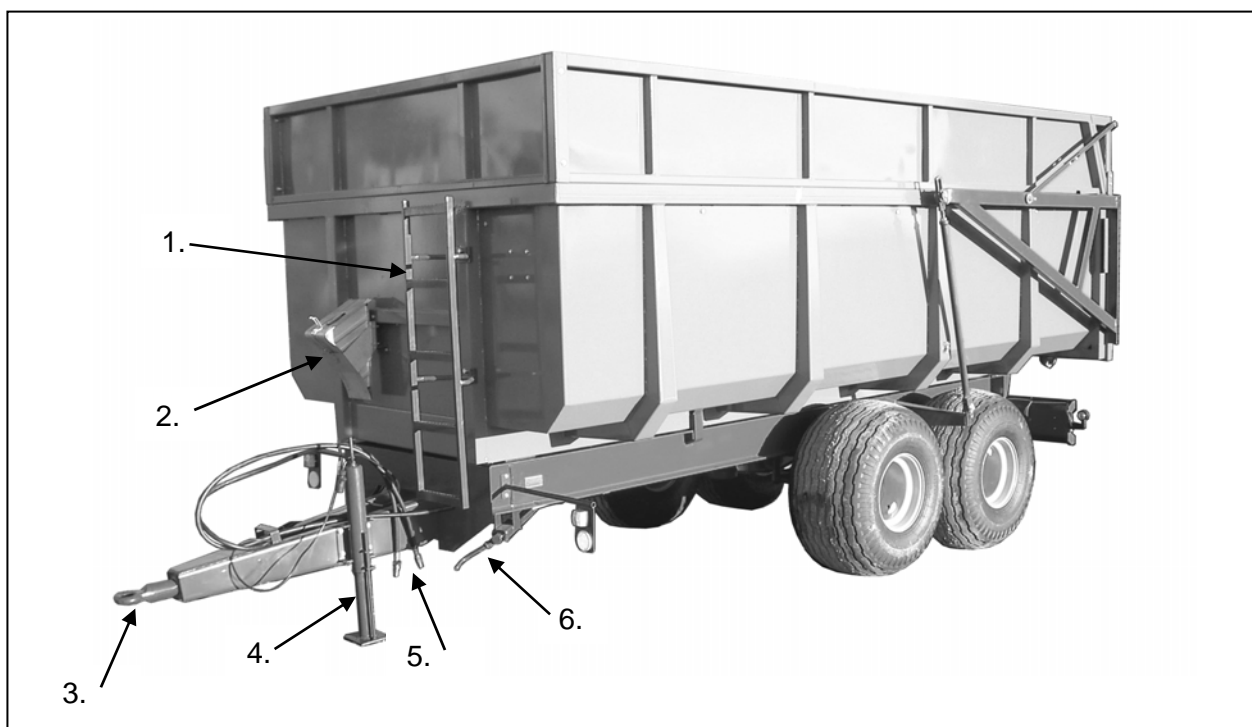
Bild 2 – Framstam och sida (bilden visar vagn med automatisk baklucka)
