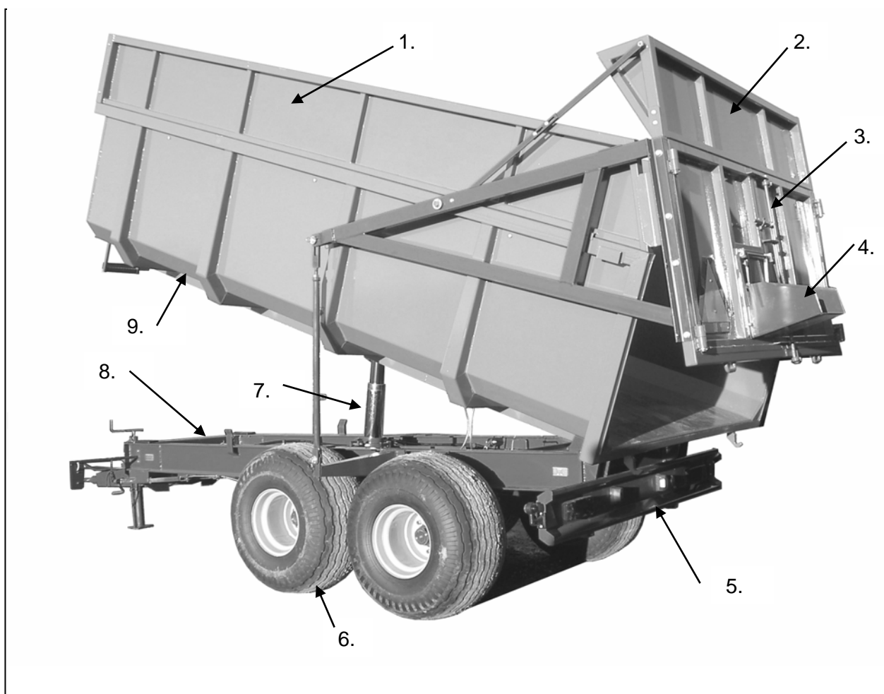
Bild 1 - Underrede och flak (bilden visar vagn med automatisk baklucka)
