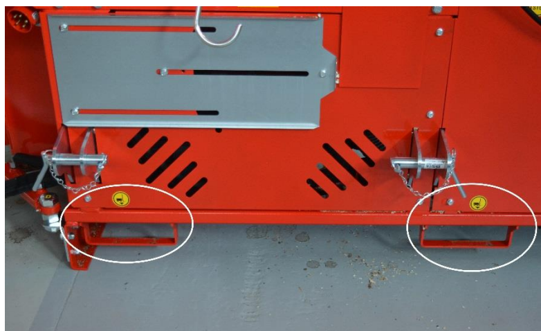
Bild 1. Maskinens lyftpunkter
