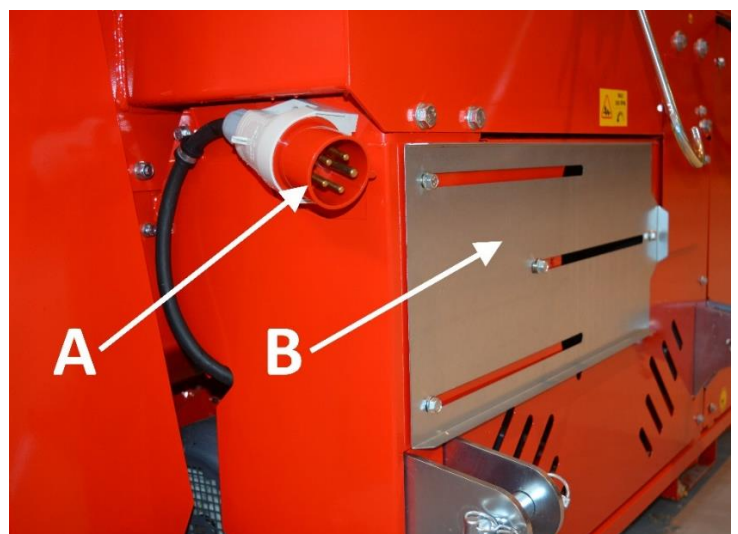
Bild 13. Maskinens elektriska drivenhet
