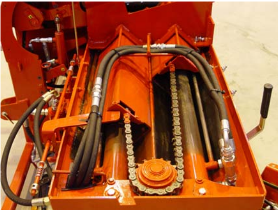
Bild 2017a (inmatningstransportören demonterad)
