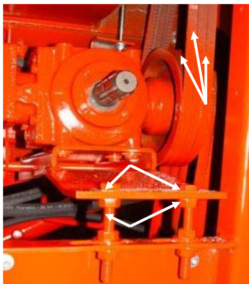
Bild 20102.7 Om du vill byta kopplings- Remmen, lossa först remmarna på vinkelväxeln
