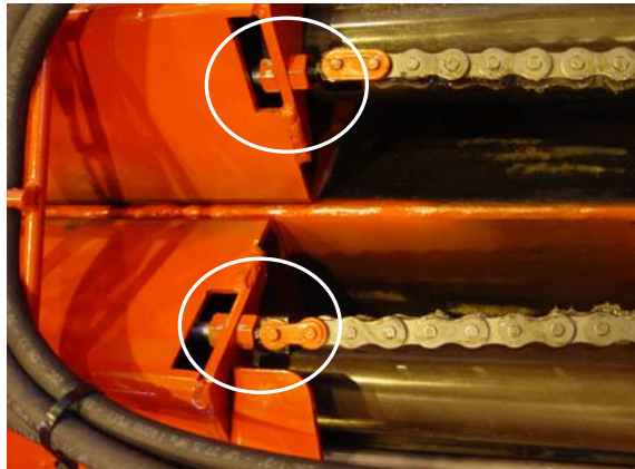
Bild 2017b (inställningspunkterna för kedjan)
