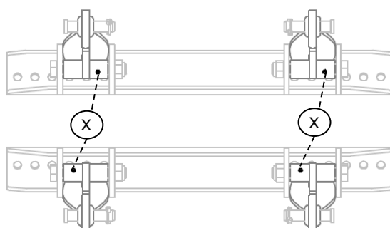
Bild.32: UPX flyttlägesfäste
