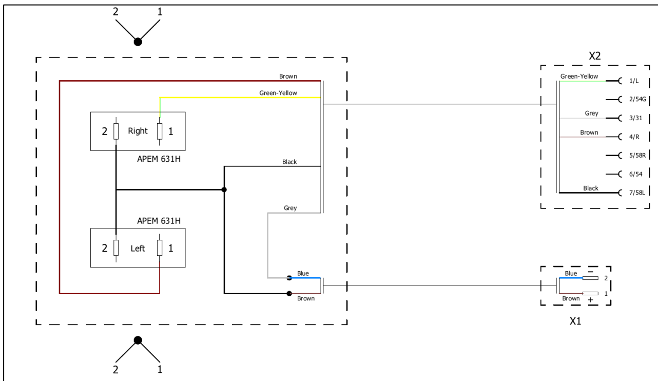
Bild.26: El-schema – kontrollbox art.nr. 330006
