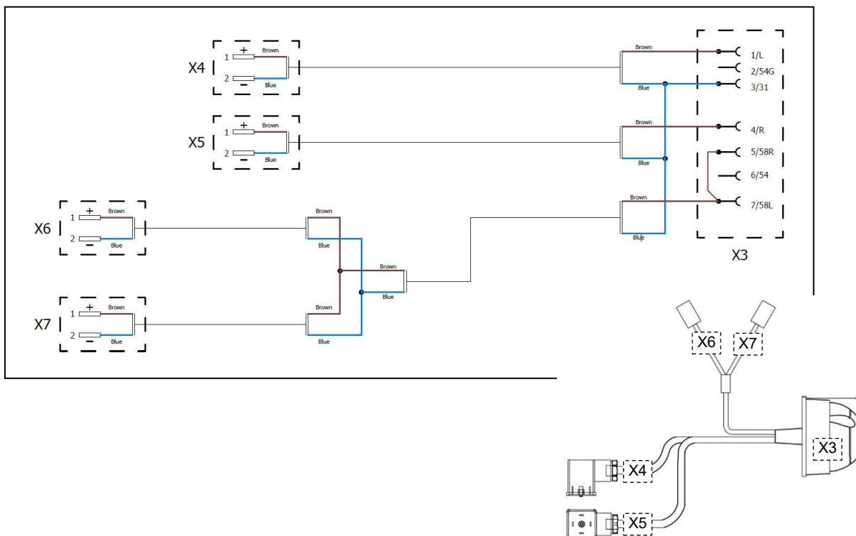
Bild.27: El-schema – kablage art.nr. 330007
