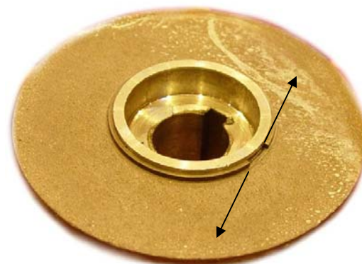
Bild 20102d Starta demontering av lamellen genom att ta bort låsringen
