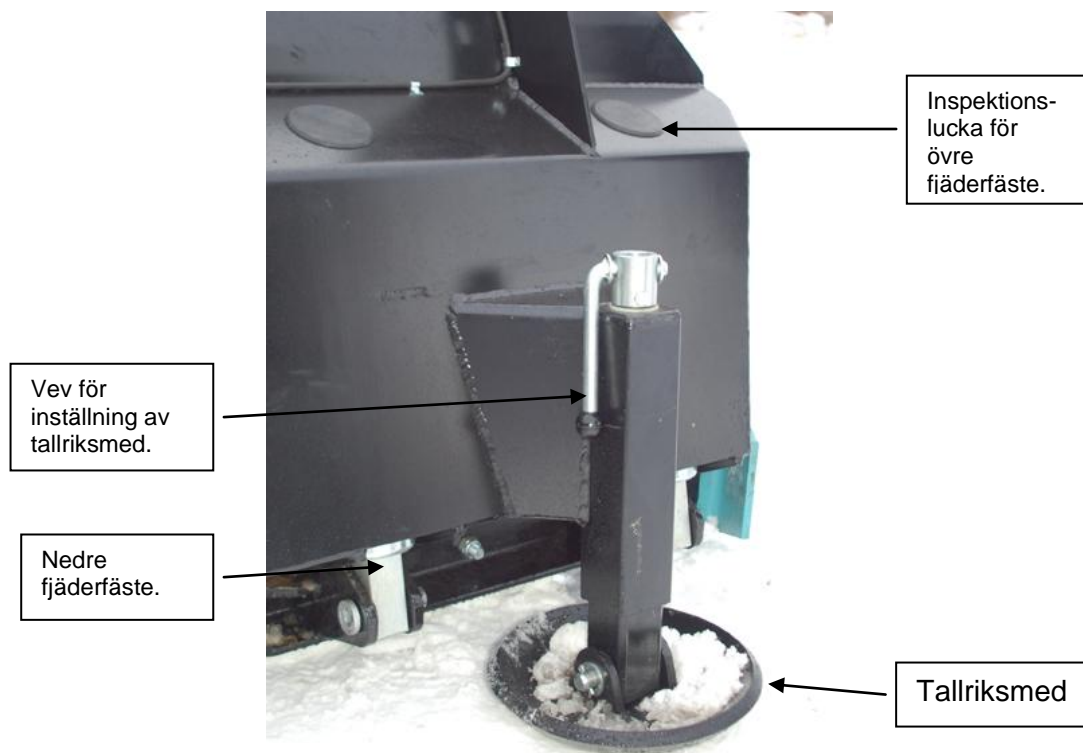
Figur 2: Översikt B
