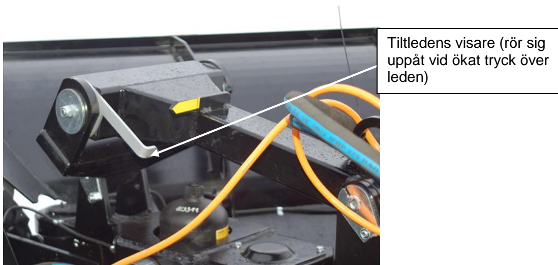
Figur 6: Visare tiltled
