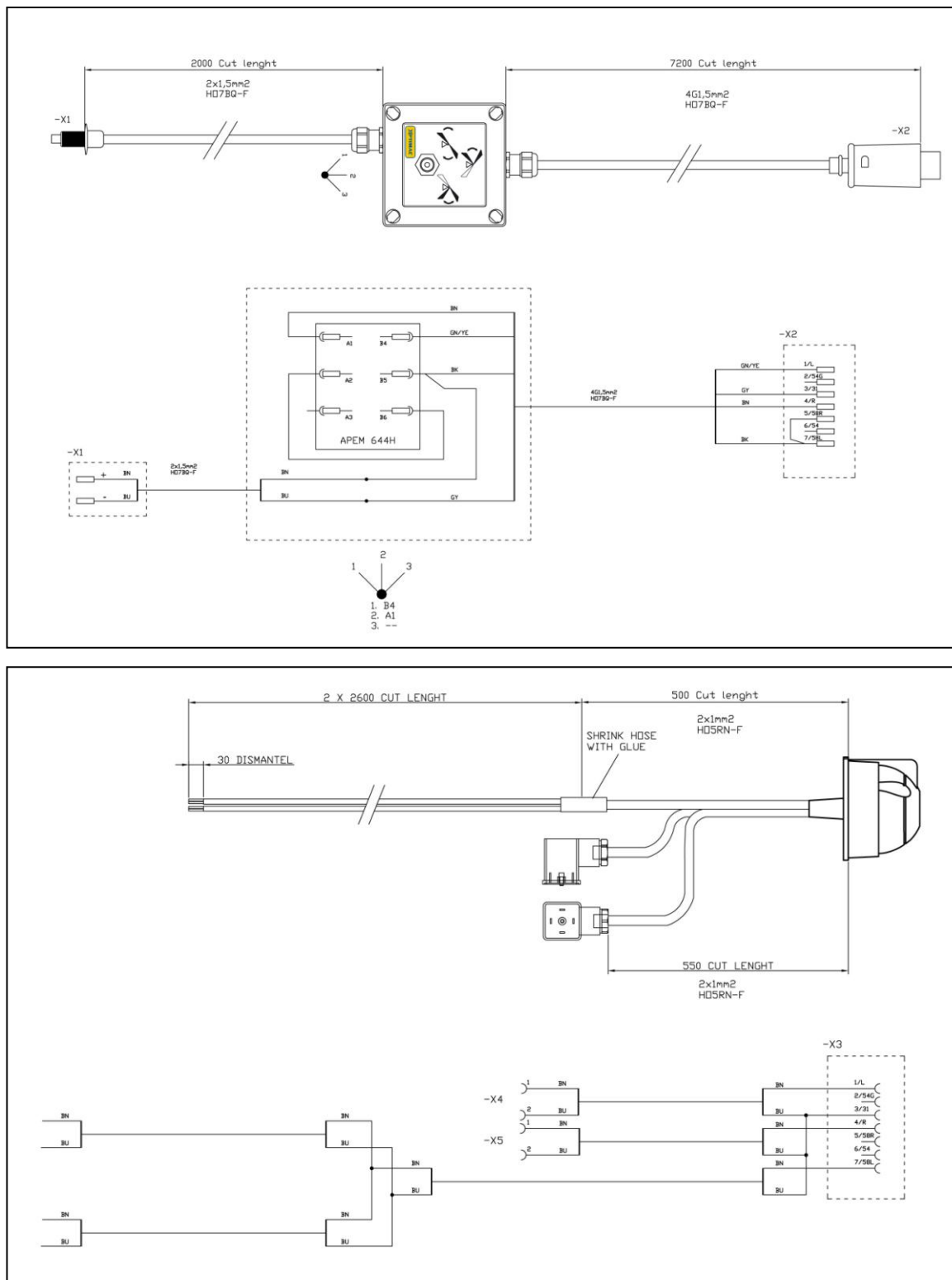
Figur 8: Elschema
