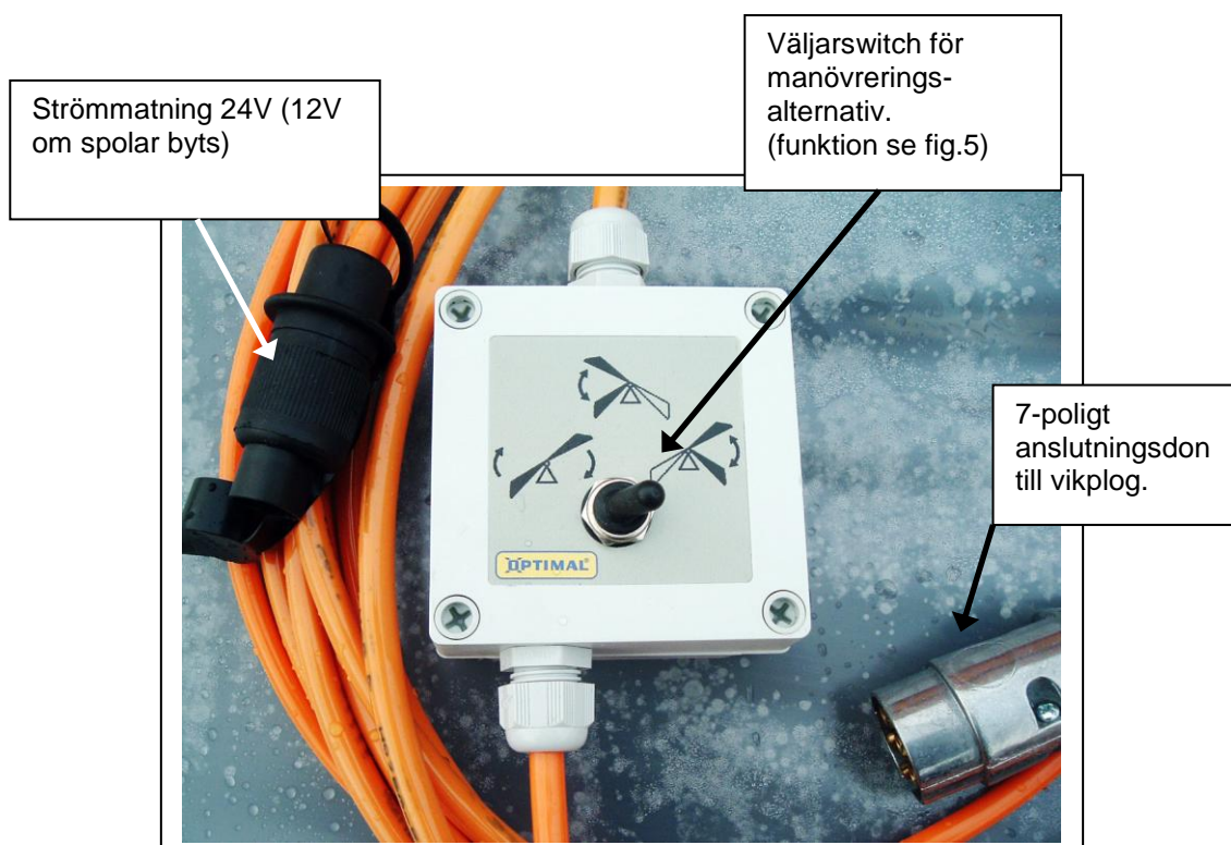
Figur 4: Handenhet
