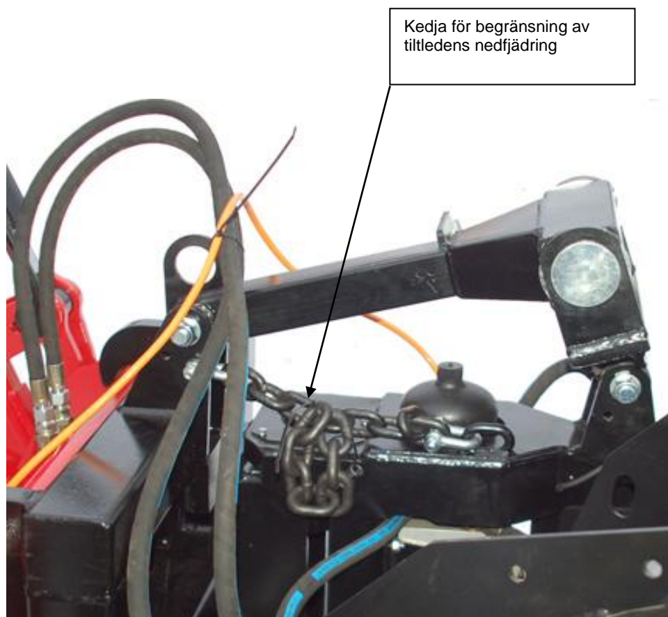
Figur 7: Begränsningskedja
